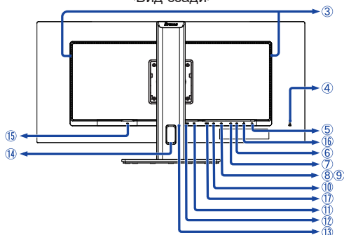
<Вид сзади>
